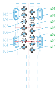
截面 2-2
