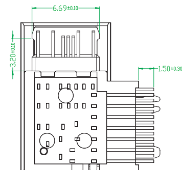
截面 3-3
