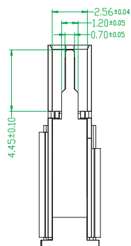
截面 2-2
